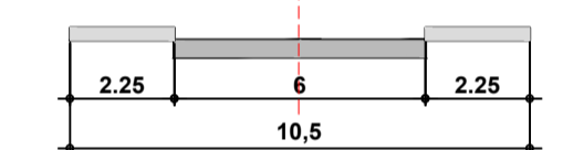
ПРЕСЕК 3 - Ул. БОЖИН НИКОЛОВ- станбена улица 1:200
